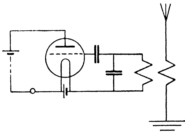
Fig. 17. De Forest's Triode Detector (1907).
