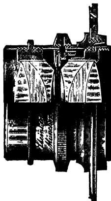
FIG. 25.—Steinheil's Orthostigmat .
