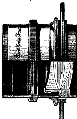
FIG. 17.—Zeiss's Anastigmat , Serie VII.
