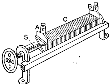
FIG. 58.—Carbon rheostat.
