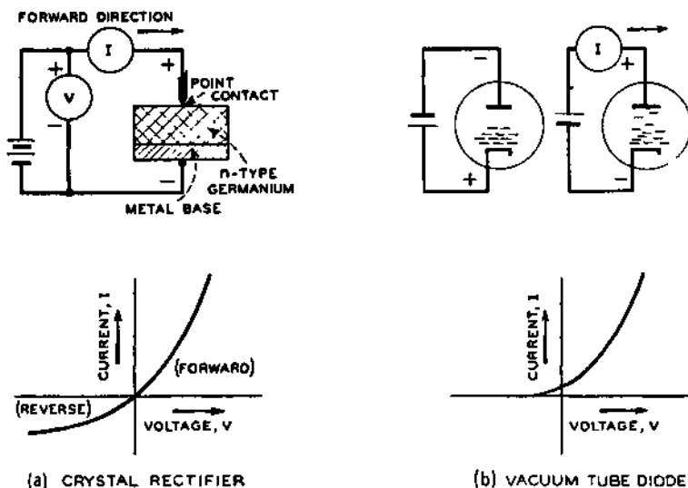
FIG. 2-1—Rectifiers and V-I Plots.
