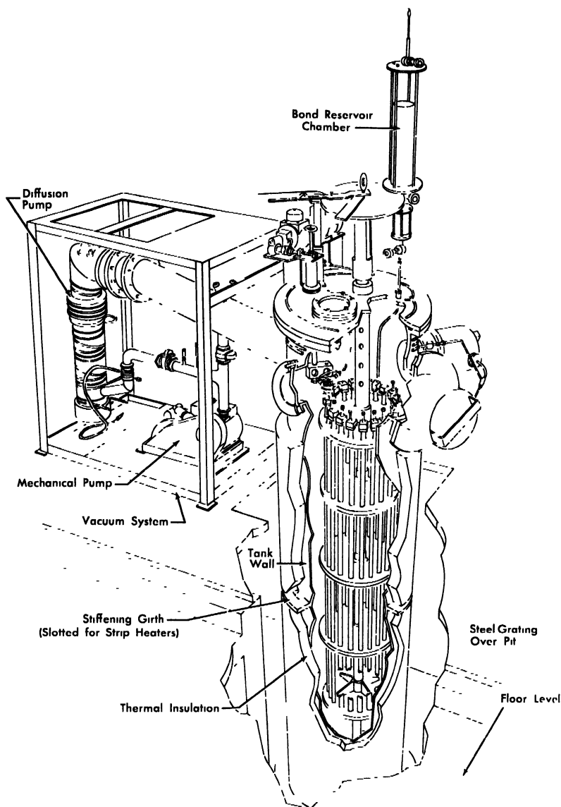
FIG. 5-10. Multirod loader
