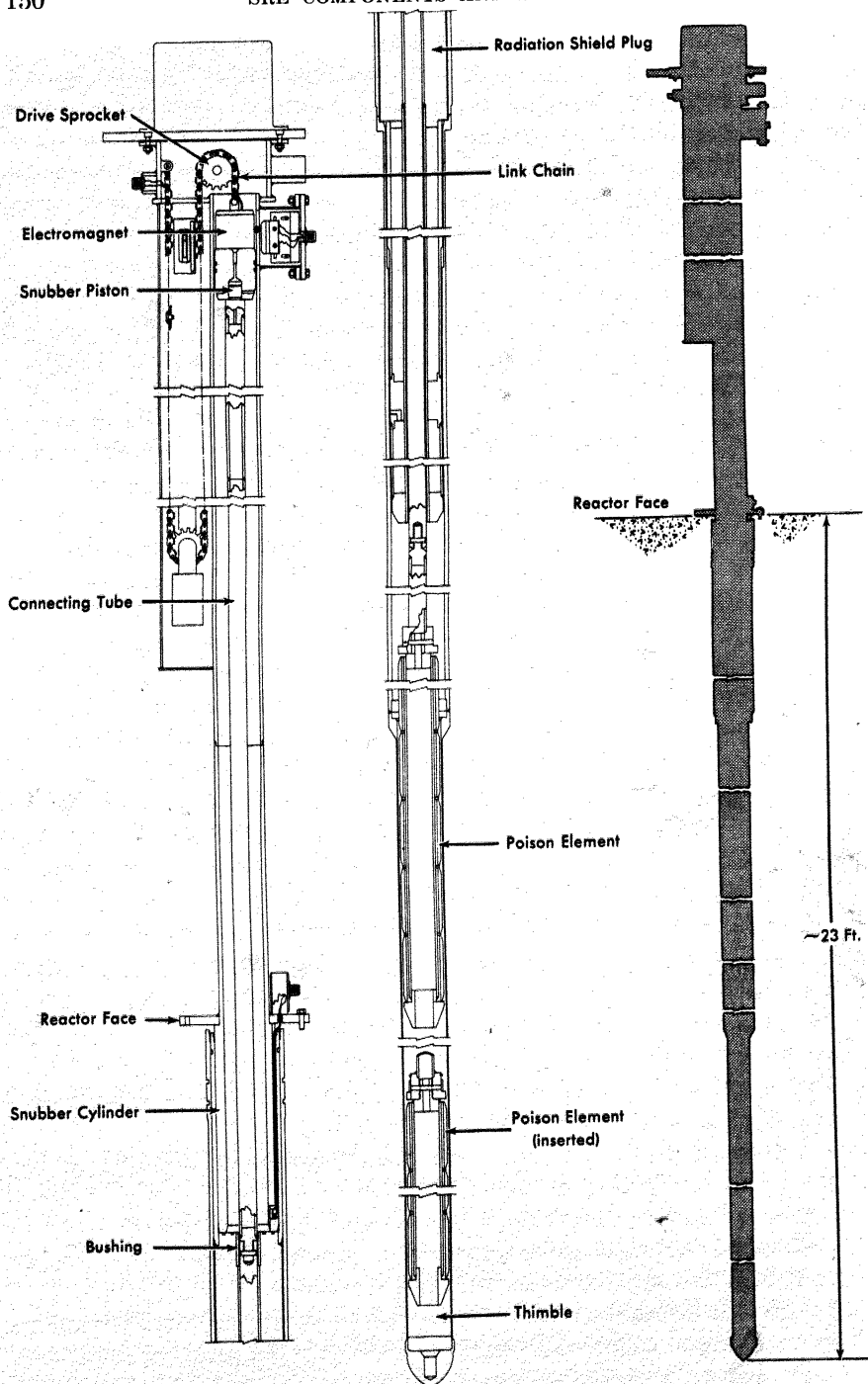
FIG. 0-9. MARK II SAFETY ROD.
