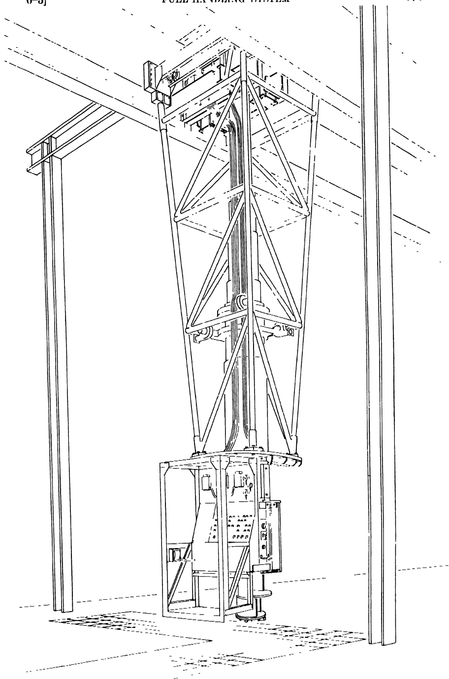
FIG. 6 20. Fuel-handling cask.
