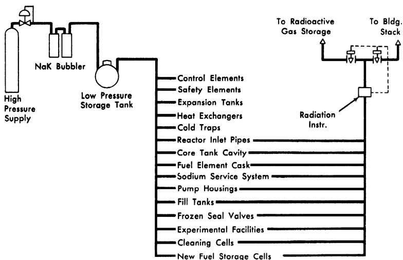
FIG. 6-23. Helium system.
