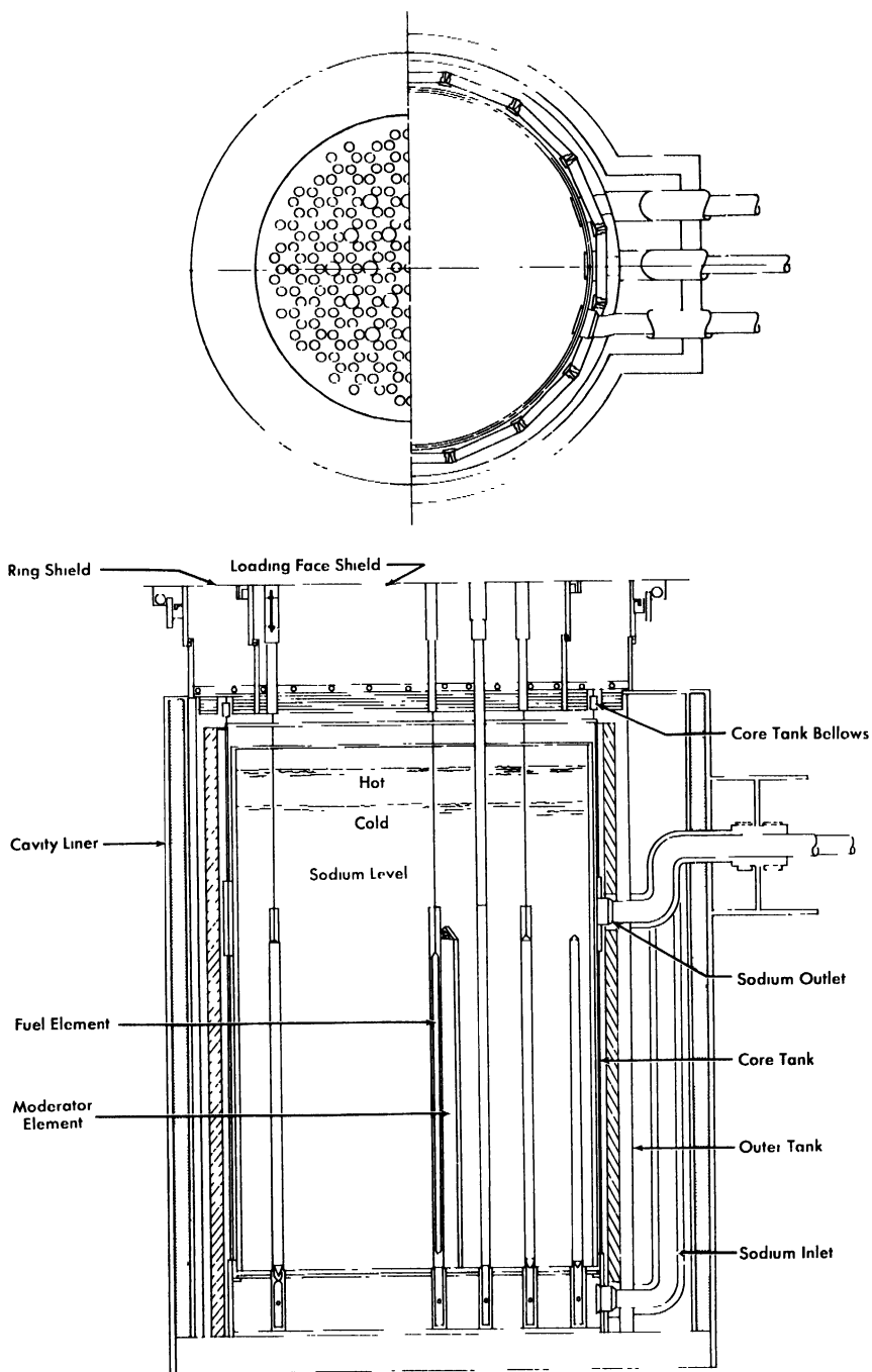
FIG. 8-8. Core, 200 Mw (electrical).
