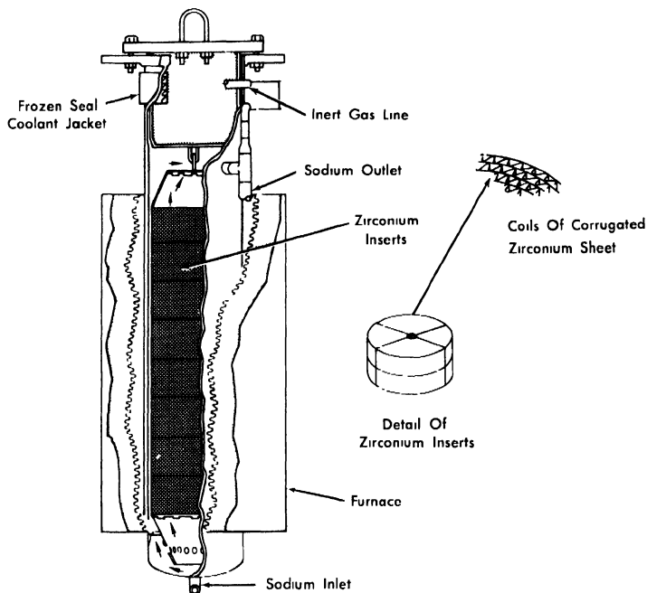
FIG. 6-18. SRE hot trap.
