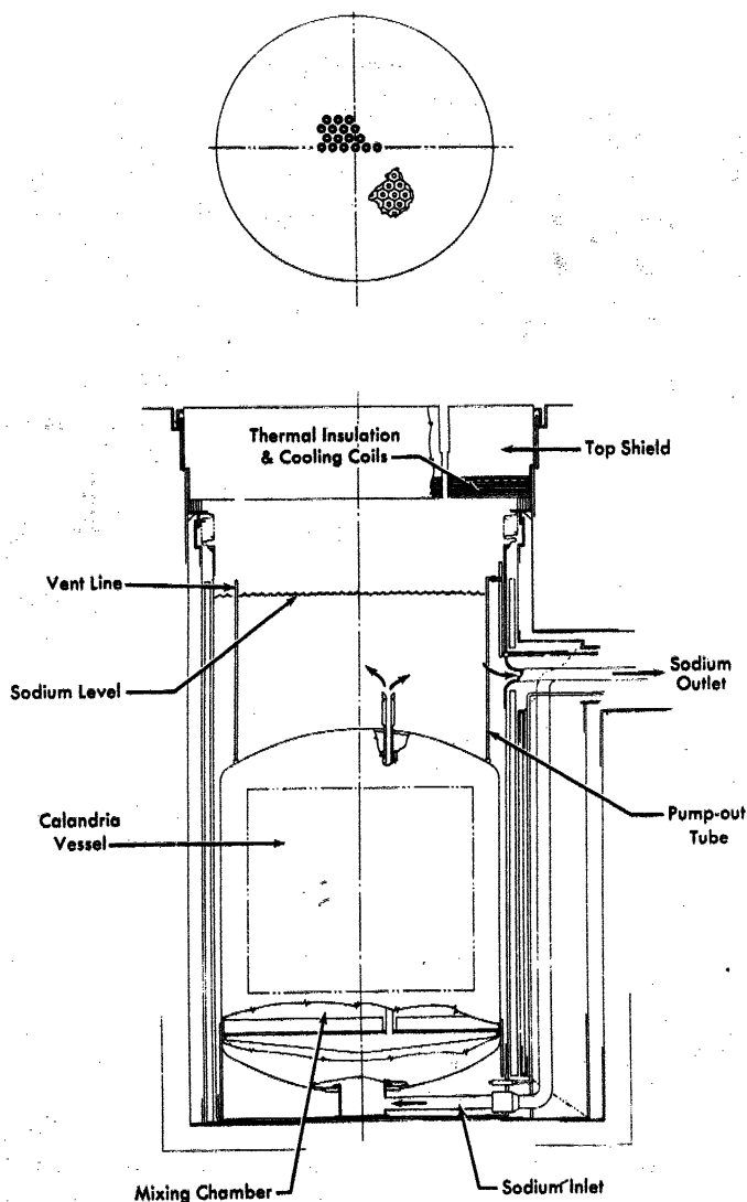
FIG. 8-9. Calandria core.
