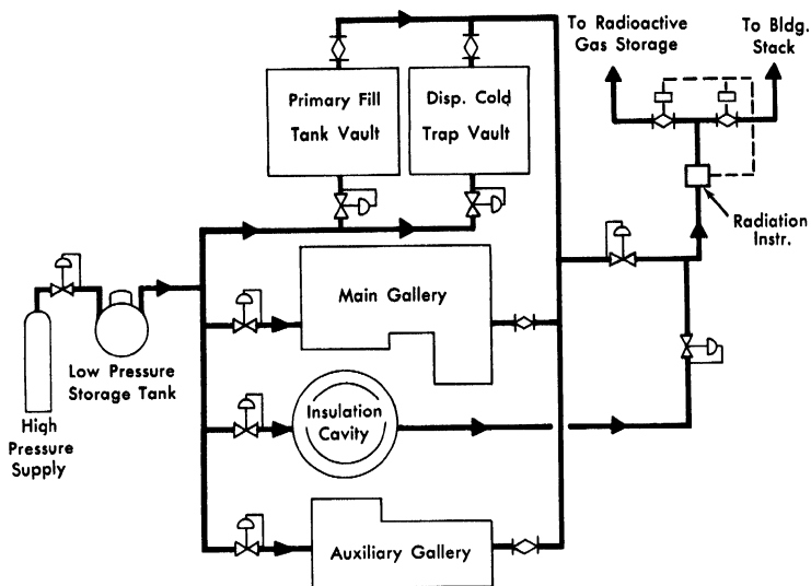
FIG. 6-24. Nitrogen system.
