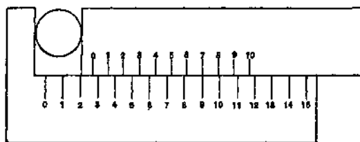
FIG. 7.—A vernier caliper.
