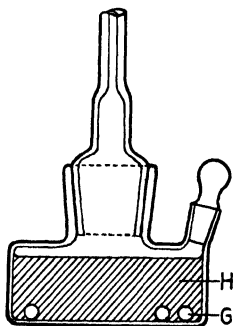
FIG. 15. Manometer vessel.
