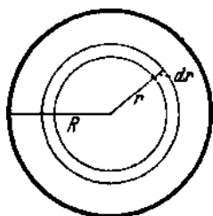
Abb. 127. Berechnung der quadratischen Momente einer Kreisscheibe.
