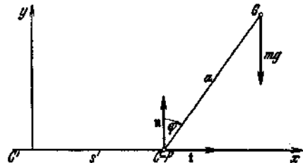
Abb. 144. Ebene Bewegung eines Körpers mit einem Stützpunkt auf einer rauhen Ebene.
