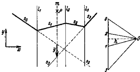
Abb. 57. Graphische Bestimmung des Moments eines ebenen Systems paralleler Kräfte.
