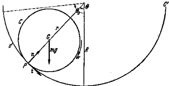
Abb. 142. Ebene Bewegung eines Rotationskörpers in einem festen Hohlzylinder.
