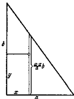
Abb. 129. Berechnung des Deviationsmoments eines rechtwinkligen Dreiecks.
