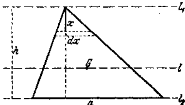
Abb. 128. Berechnung der quadratischen Momente eines Dreiecks.
