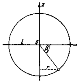
Abb. 117. Zum sphärischen Pendel.
