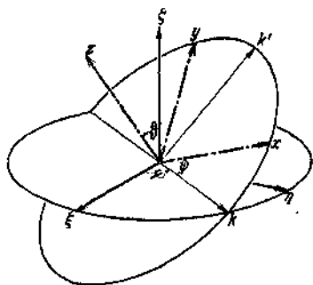
Abb. 135. Die Eulerschen Winkel.
