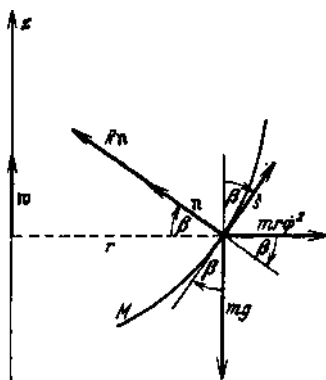
Abb. 116. Bewegung eines schweren Massenpunktes auf einer Rotationsfläche.
