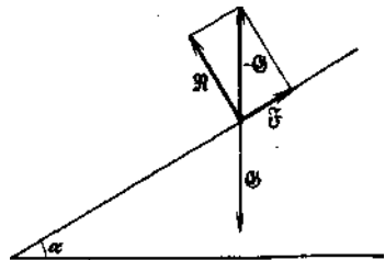
Abb. 16. Gleichgewicht eines Massenpunktes auf einer rauen schiefen Ebene.
