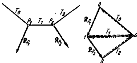
Abb. 45. Kräftediagramm eines Stabpolygons.
