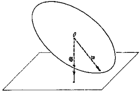
Abb. 134. Trägheitsellipsoid, Drehvektor und Moment der Bewegungsmenge.
