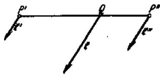
Abb. 42. Verlegung der Kräfte in die Knotenpunkte.
