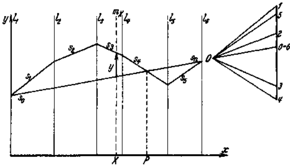
Abb. 58. Graphische Bestimmung von Schubkraft und Biegemoment eines querbelasteten Balkens.
