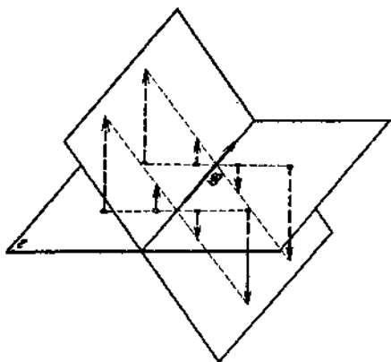
Abb. 33. Momentebene eines ebenen Vektorsystems.
