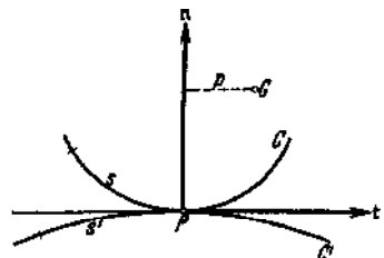
Abb. 140. Rollen und Gleiten.
