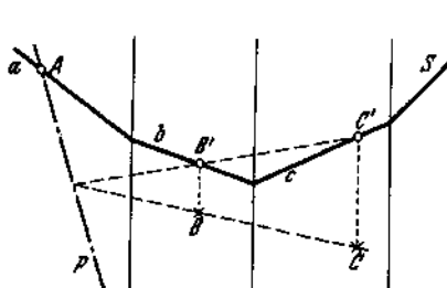
Abb. 55. Konstruktion eines Seilpolygons für parallele Kräfte, von dem drei Seiten durch vorgeschriebene Punkte gehen.
