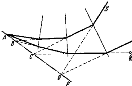
Abb. 52. Polarachse von zwei Seilpolygonen.
