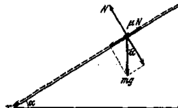
Abb. 98. Bewegung eines schweren Massenpunktes auf einer rauhen schiefen Ebene.
