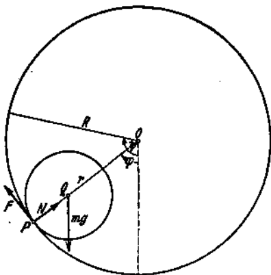
Abb. 146. In einem drehbaren Hohlzylinder rollender Rotationskörper.
