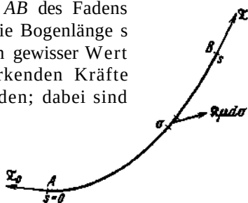
Abb. 159. Gleichgewicht eines Fadens.
