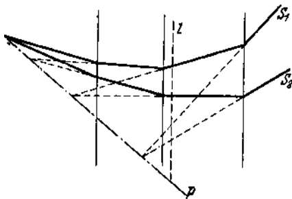
Abb. 54. Affinität zweier Seilpolygone für parallele Kräfte.
