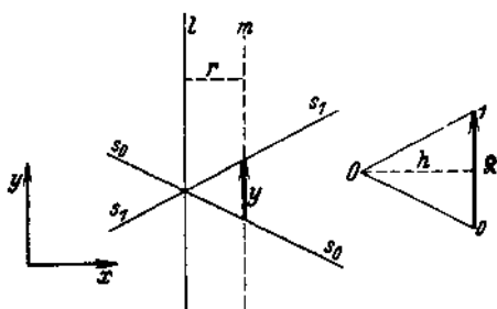
Abb. 56. Graphische Bestimmung des Moments einer Kraft.
