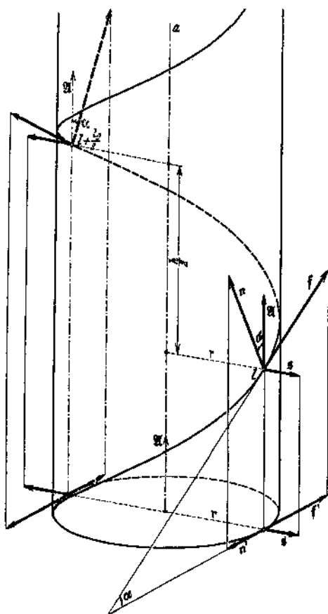
Abb. 39. Reaktionen einer festgehaltenen Schraubenlinie.
