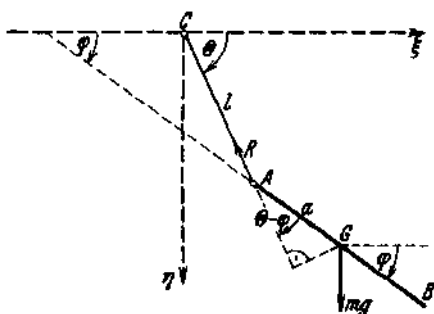
Abb. 139. Ebene Bewegung eines an einem Faden aufgehängten Stabes.
