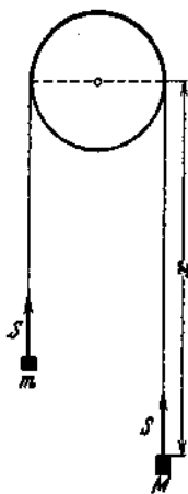
Abb 100. ATWOODSche Fallmaschine.
