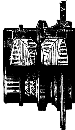
FIG. 25.—Steinheil's Orthostigmat .
