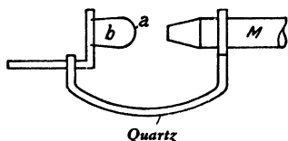
FIG. 11.—Loop electrometer (Kolhorster).
