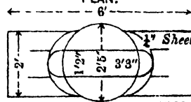
DAMPER Fig. 10.
