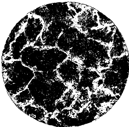
चित्र ६३—१.४% कार्बन इस्पात
