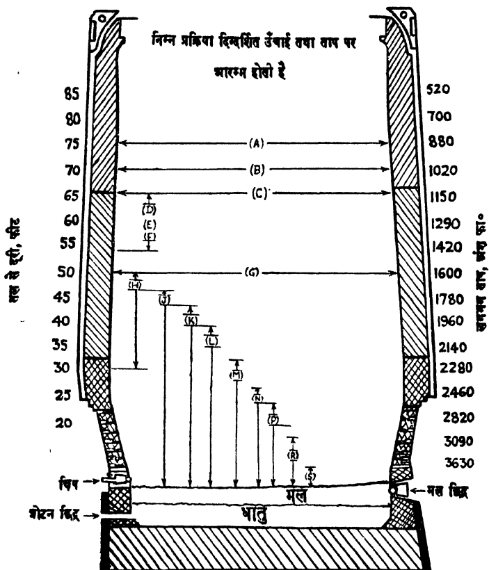
चित्र १५—प्रवात फर्नेस के विभिन्न प्रक्रिया क्षेत्र
