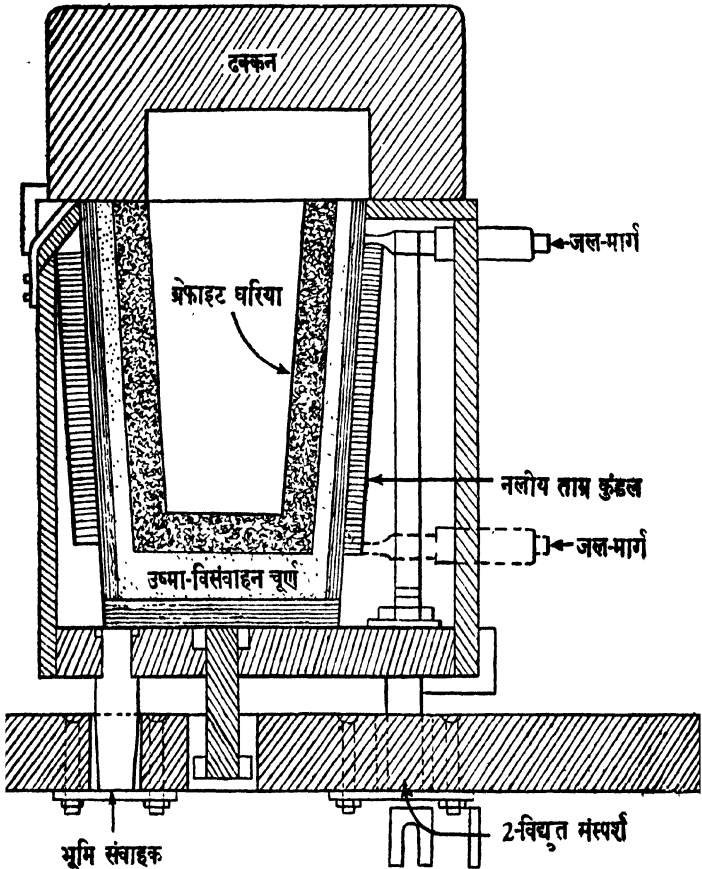
चित्र २८ क—विद्युत-उष्म प्रेरक फर्नेस
