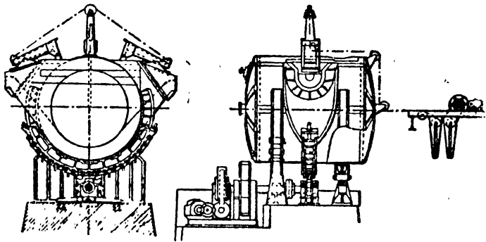
चित्र ३६—गरम धातु-मिश्रक
