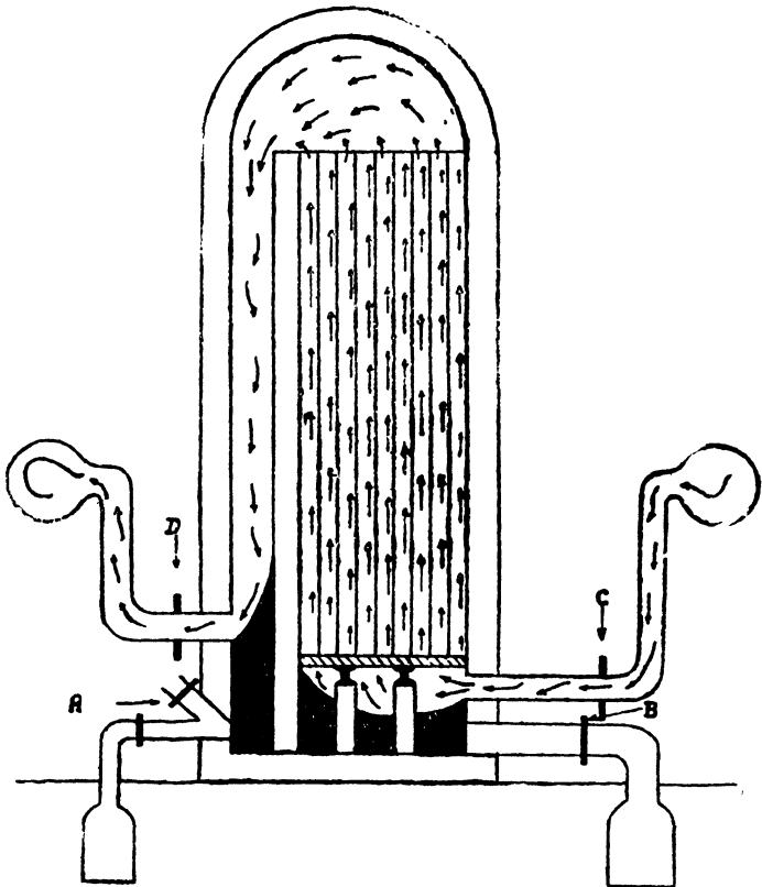
चित्र १३ ख—उष्ण प्रवात स्टोव (हवा पर)
