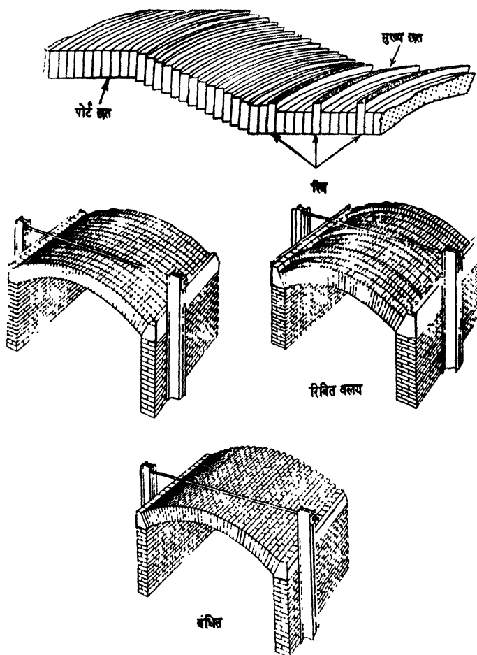
चित्र ४४—विद्युत तंबूर फर्नेसों की छतों में ईंटों सज्जित करने के विविध तरीके
