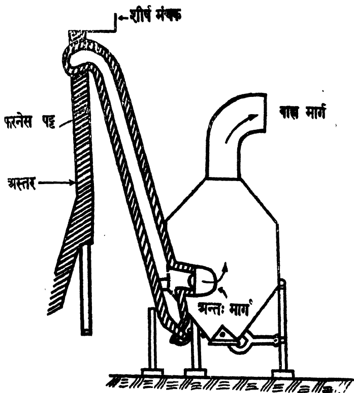
चित्र १४—धूलिधारक का कार्यकारी सिद्धान्त
