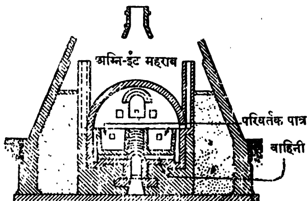
चित्र २२—सीमेण्टन फरनेस
