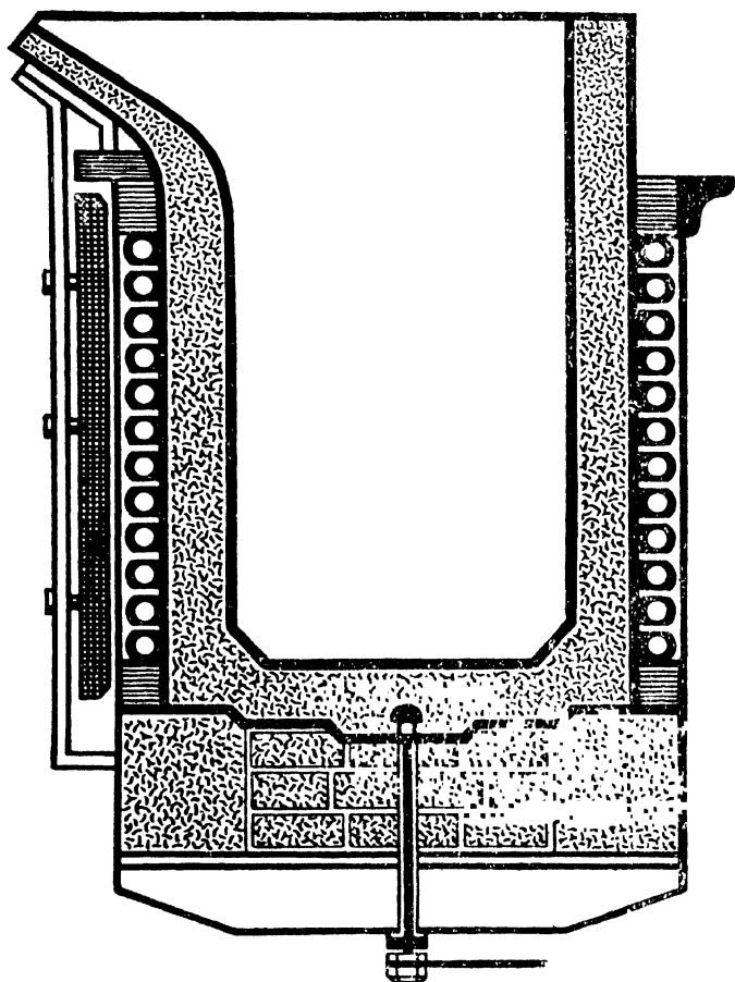
चित्र ५४ क—विद्युत प्रेरक फर्नेस की मुख्य बनावट
