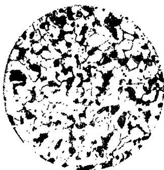
चित्र ५ एफ—०.४ प्रतिशत कार्बन इस्पात
