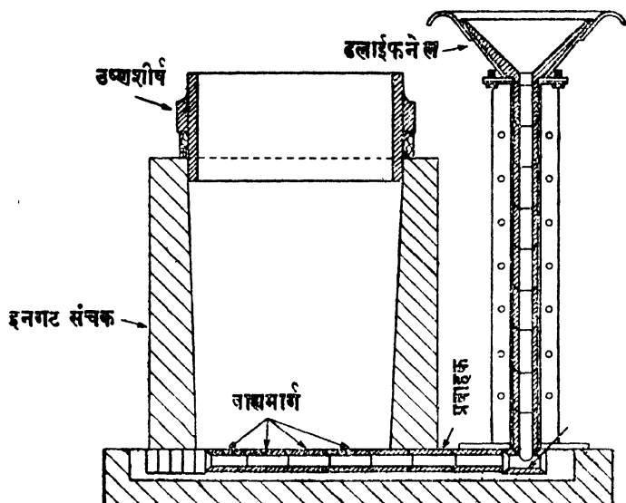
चित्र ५६—इस्पात के नितल प्रपूरण की विधि
