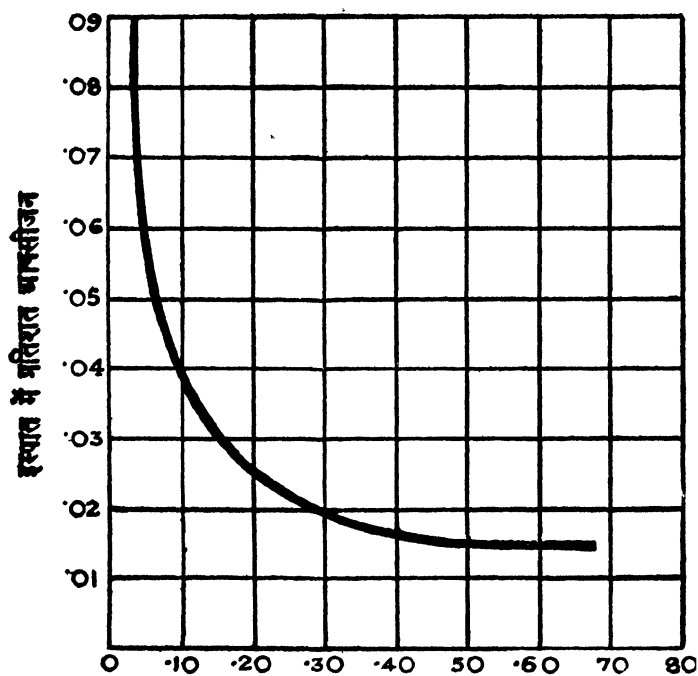
इस्पात में प्रतिशत कार्बन
