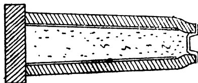
चित्र ५८ — इस्पात प्रपूरण के लिए उपयुक्त विविध मोल्ड
