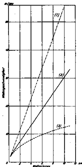
Fig. 4. Wellengeschwindigkeit an einer Grenzfläche mit ca. 5.4^\circ Temperatursprung; (1) bei isothermer Schichtung, ohne Zustandsänderung, (2) bei isothermer Schichtung und adiabatischer Zustandsänderung, (3) bei konstanter Dichte in jeder Schicht.
