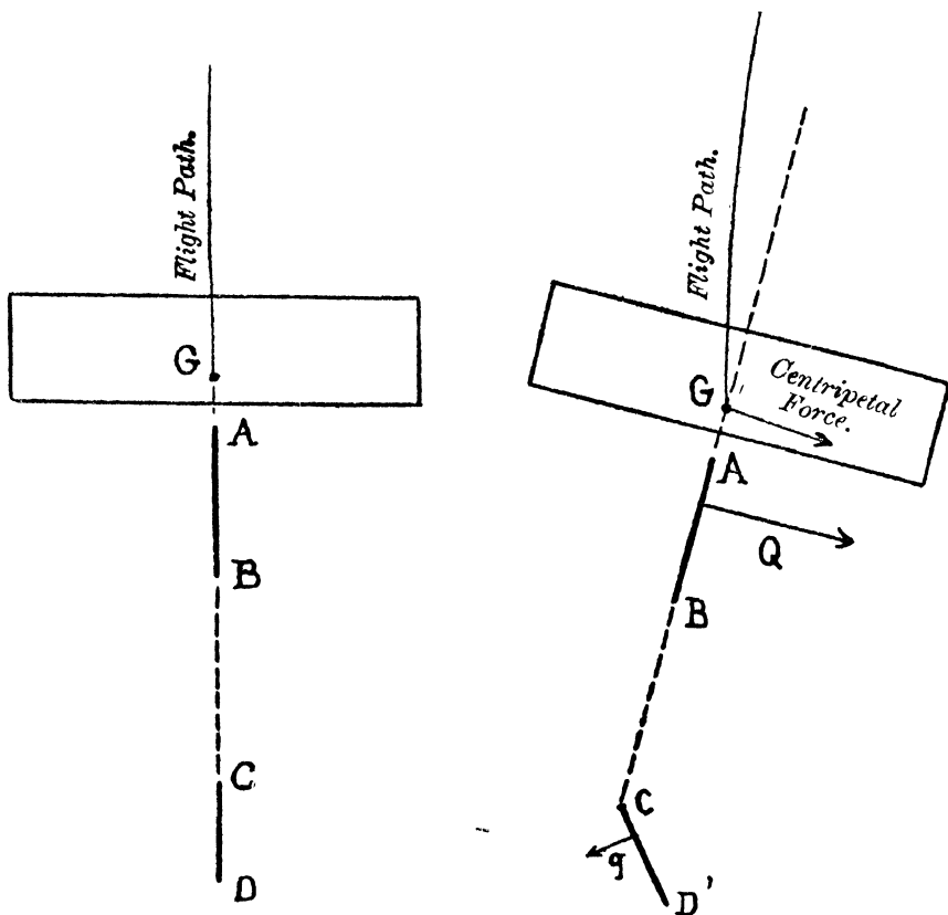
FIG. 77.—Plan.
