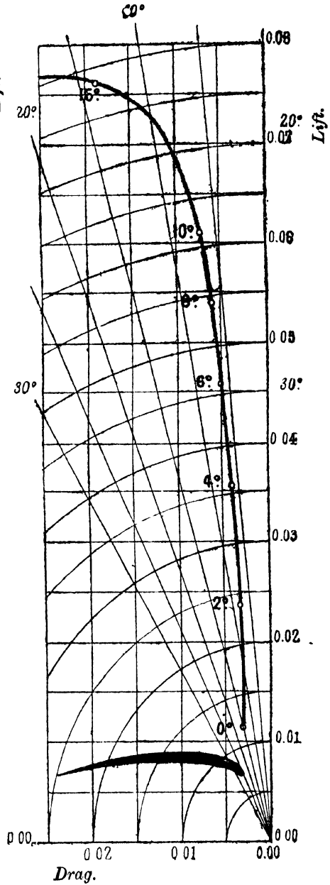
FIG. 4.—Bleriot XI. plane.
