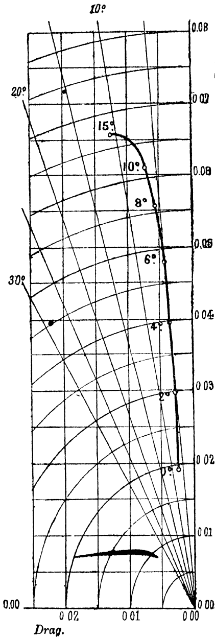
FIG. 3.—Bréguet plane.
