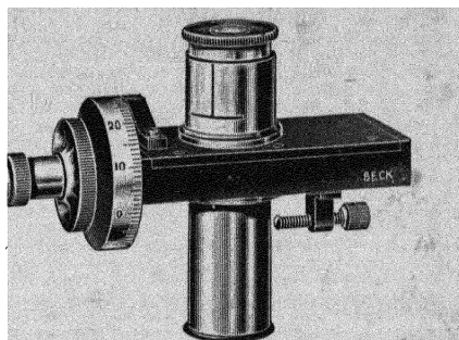
FIG. 55. COBWEB EYEPIECE MICROMETER (Beck)
