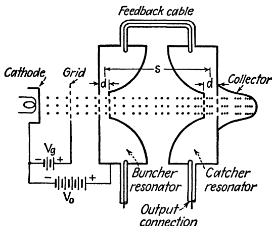
FIG. 10.—Klystron oscillator.
