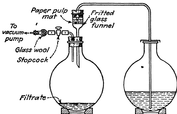
FIG. 5. Filtering apparatus.
