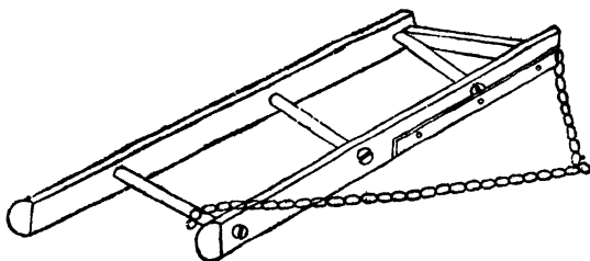
Fig. 45. Split log drag
