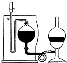
Fig. 68.—Explosion pipette.
