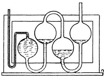
Fig. 69.—Double pipette.
