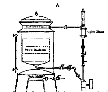
FIG. 76.—Extraction Apparatus.
