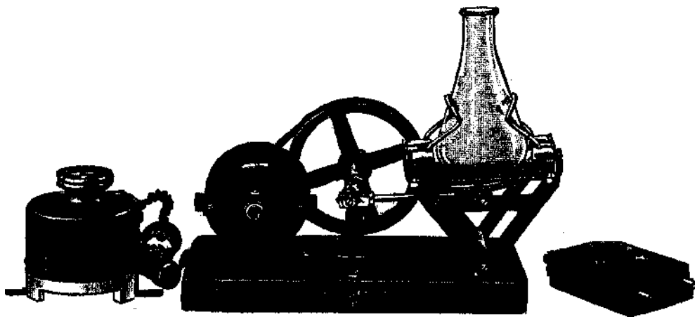
FIG. 55.—Shaking Apparatus
