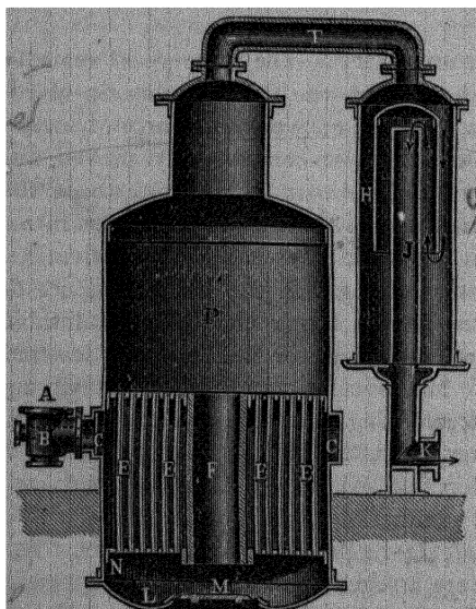
FIG. 45.—Vacuum-pan.
