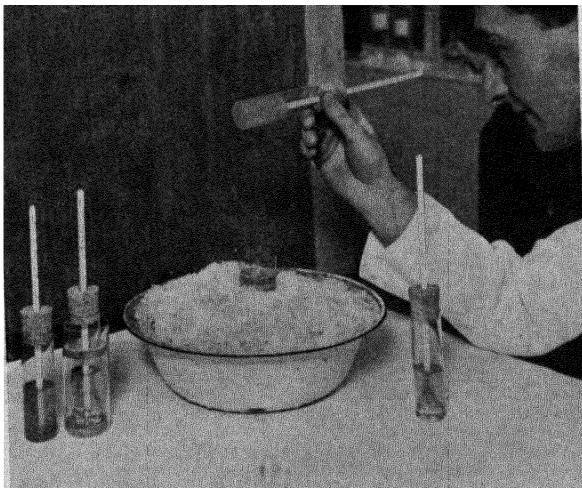
Fig. 5.—POUR POINT TEST.
