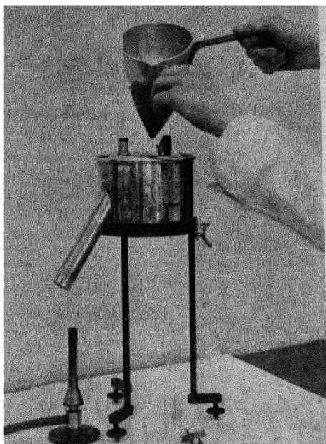
Fig. 2.—REDWOOD VISCOSITY (2).
