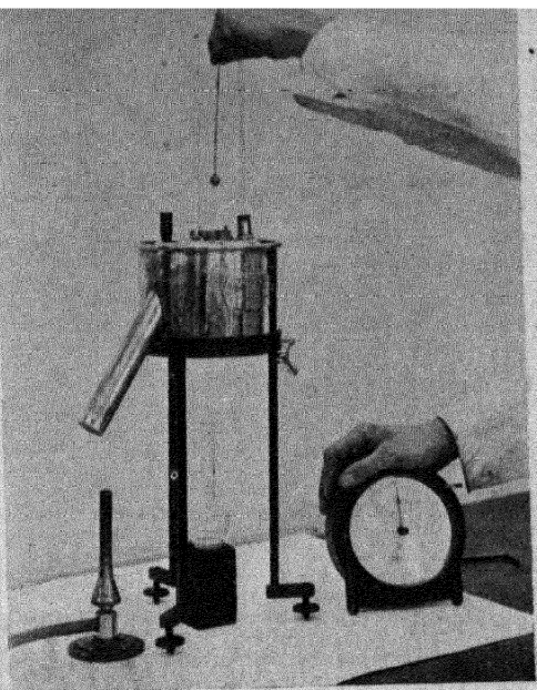
Fig. 3.—REDWOOD VISCOSITY (3).
