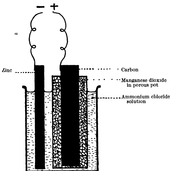
FIG 4—Leclanché cell.
