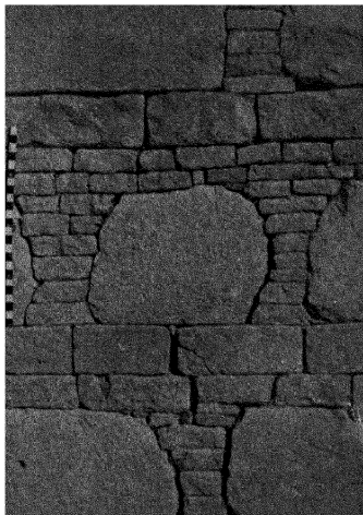
4. SEMI-ASHLAR.
