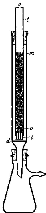
Abb. 7. Adsorptions-Vorrichtung nach DHERE und VEGEZZI (Zeichnung bei VEGEZZI).
