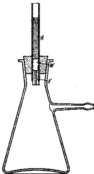
Abb. 24. Adsorptionsrohr aus Quarz (montiert).
