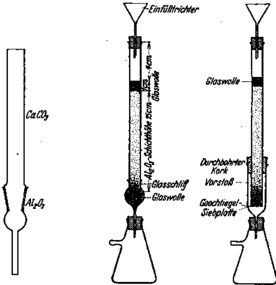
Abb. 12. Adsorptionsrohr nach KÜHN und BROCKMANN, für analytische Zwecke.
