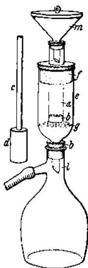
Abb. 6. Apparat von DHERE und ROGOWSKI (Zeichnung bei ROGOWSKI). Rohr 25 \times 2 cm, Füllhöhe 6–8 cm. Auf dem Korkstopfen Filterpapier, darüber 1–2 cm Sand. — Links Holzpistill.
