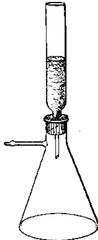
Abb. 4. Einfache Adsorptionsvorrichtung.
