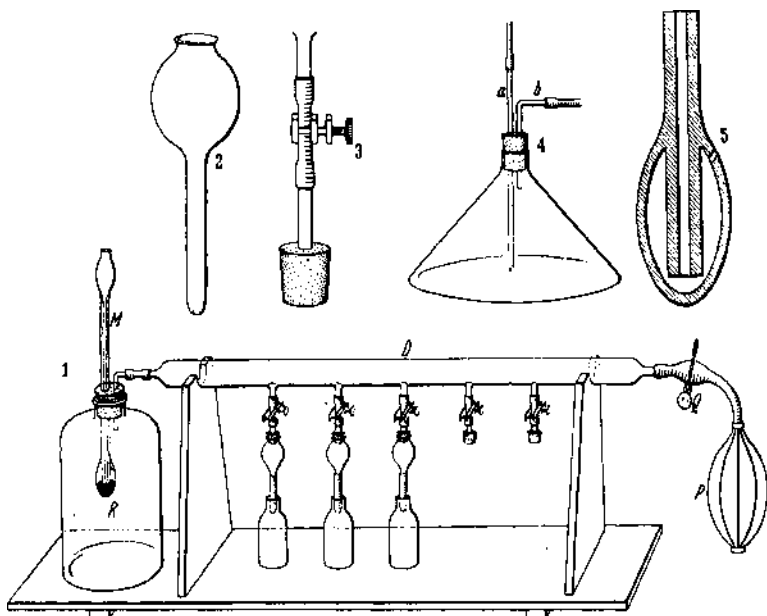
Abb. 2. Originalvorrichtung von TSWETT.
