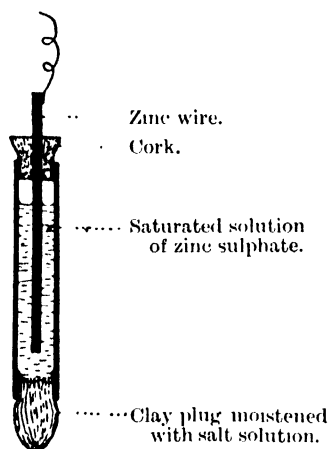
FIG. 7.—Non-polarisable electrode.
