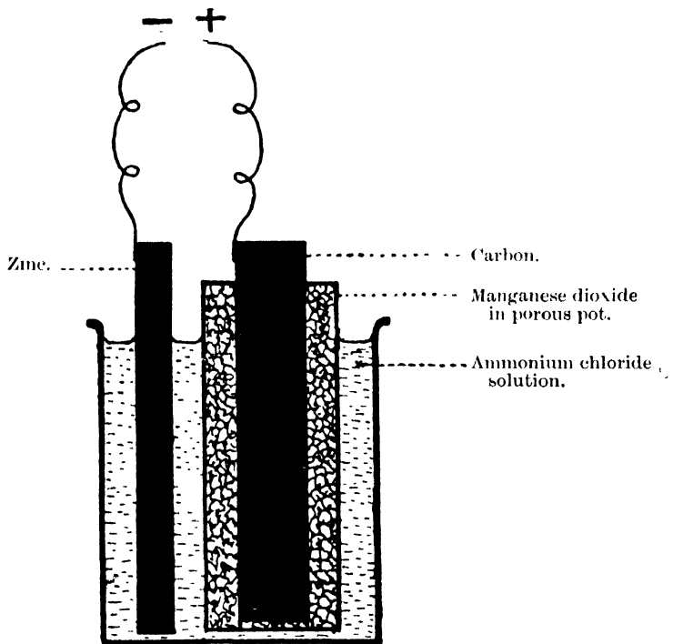
FIG. 4.—Leclanché cell.
