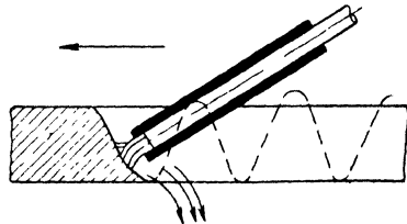
Fig. 116. Metal-arc cutting
