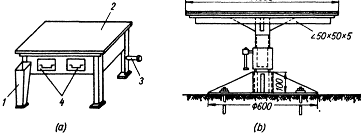
Fig. 30. Welding tables
