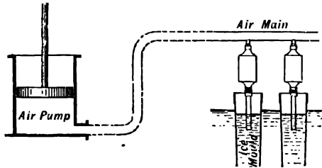
Fig. 41. Pneumatic Agitator.
