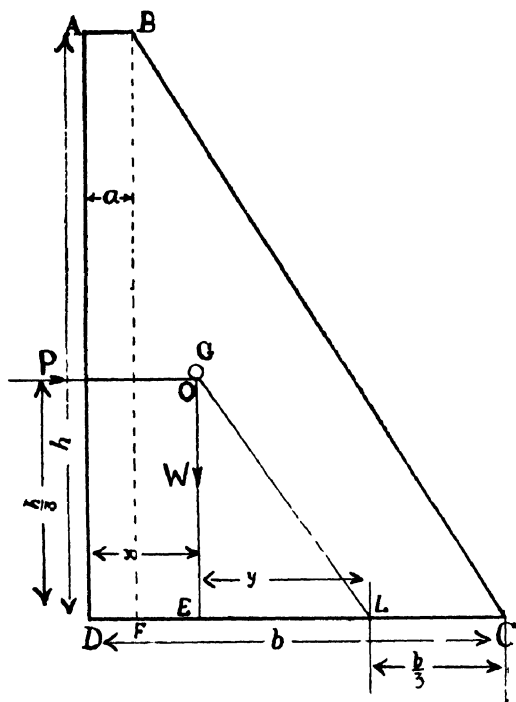
Fig. 179.—Trapezoidal Dam.
