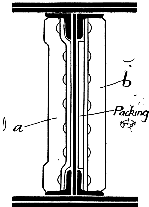
Fig. 267.—Stiffeners.
