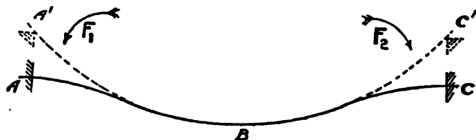
Fig. 94.—Fixed Beams.
