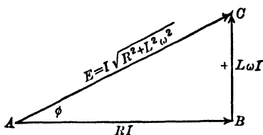
FIG. 137.—E.m.f. diagram.
