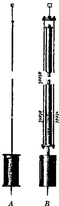
FIG. 24. Compensation Pendulums
