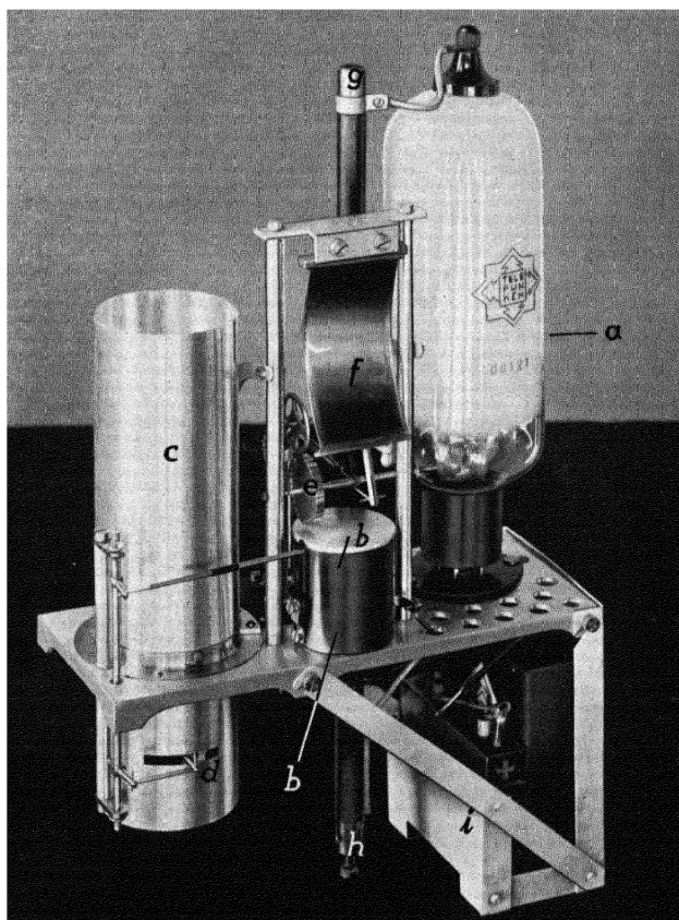
Abb. 3. Radiofonde Dufort-Telefunken ohne Schutzkappe mit Batterien.
