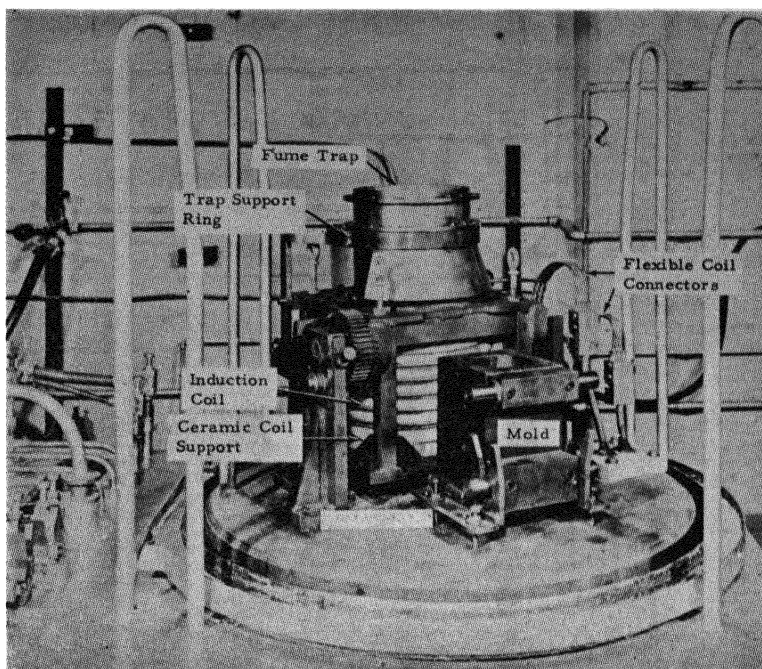
Fig. 9—Furnace Interior.
