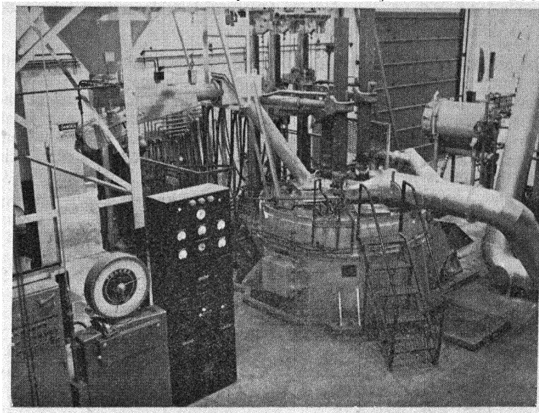
Fig. 2—1500 KW 3 Phase Ore Melting Furnace
