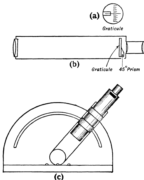
Fig. 82.—Auto-collimator
