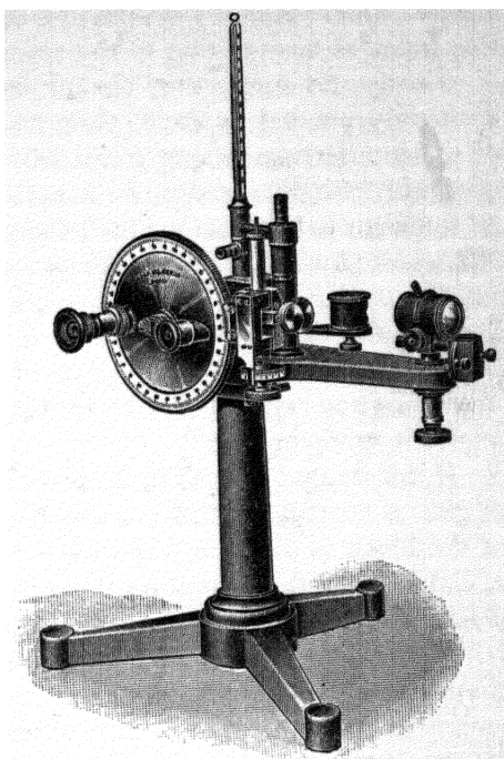
Fig. 87.—Pulfrich Refractometer
