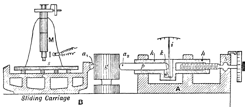
Fig. 28.—Société Gènevoise Measuring Machine (diagrammatic)
