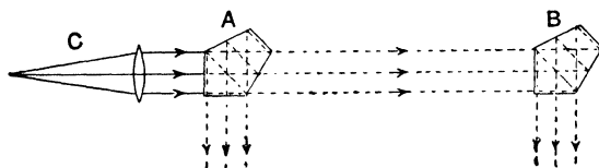
Fig. 73b.—The König Adjuster
