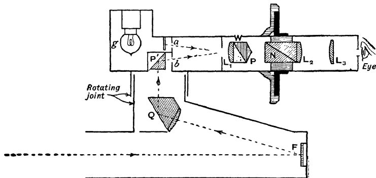
Fig. 145.—König-Martens Illumination Photometer
