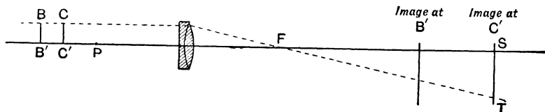
Fig. 37.—Tacheometry
