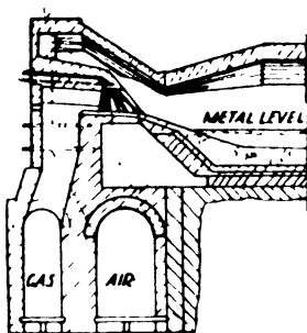
FIG. 77. Venturi port.
