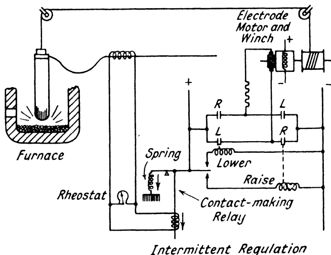
FIG. 116. Electrode-control diagram.
