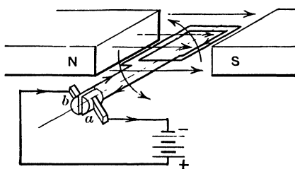
FIG. 79.—Simple Motor.
