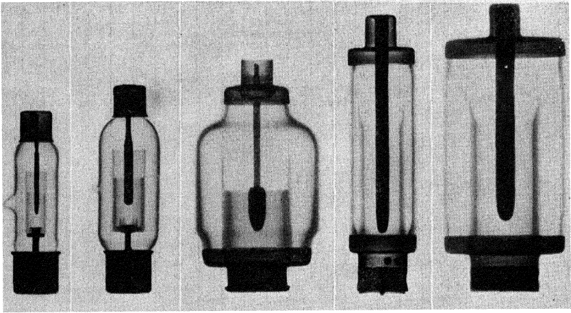
(a) 1B29. (b) 1B22. (c) 1B31. (d) WX3226. (e) WX3240.
