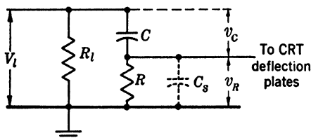
FIG. A-17.—Differentiating RC -circuit.
