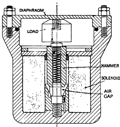
Fig. 14.—Diaphragm Sounder
