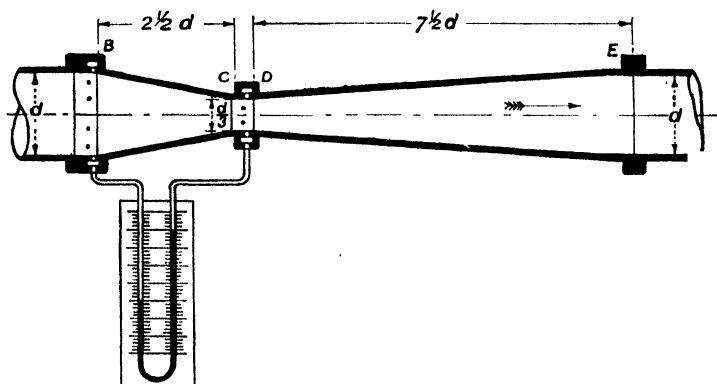
Fig. 11.—Venturi Meter.
