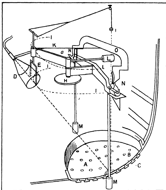
Fig. 22.—Walser Apparatus
