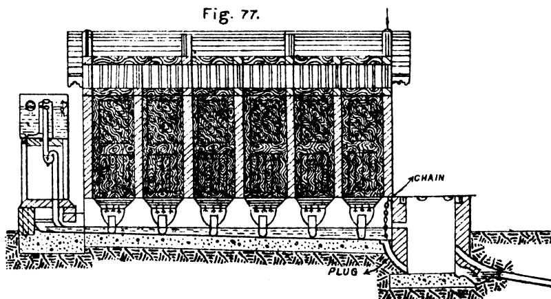
LONGITUDINAL SECTION.
