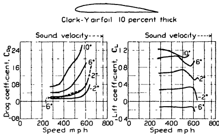
FIG. 128. Compressibility effect. (N.A.C.A.)
