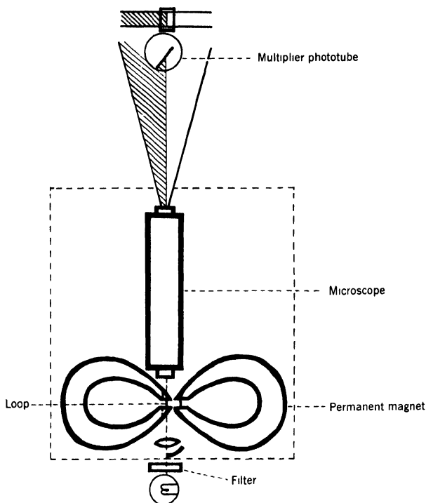
Fig. 1.2. Photoelectric amplifier.
