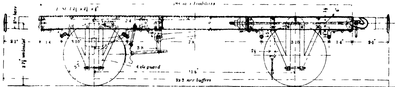
ELEVATION
