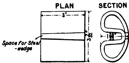
FIG. 21. STUARTS PATENT KEY
