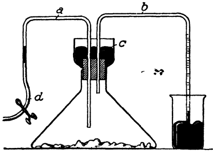
FIG. 8.—Kostychev's flask.
