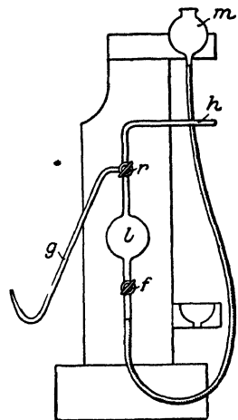
FIG. 9.—Kostychev's gas pipette.
