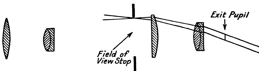
FIG. 23A. KELLNER EYEPIECE
