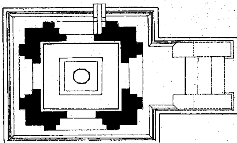
PAVAR : PLAN OF TEMPLE.
