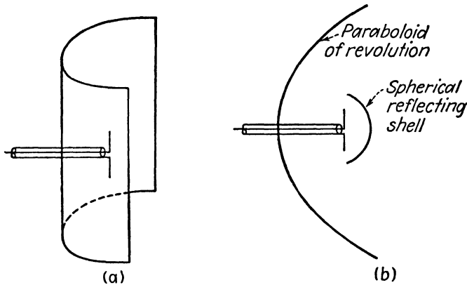
FIG. 19.—Parabolic antennas.
