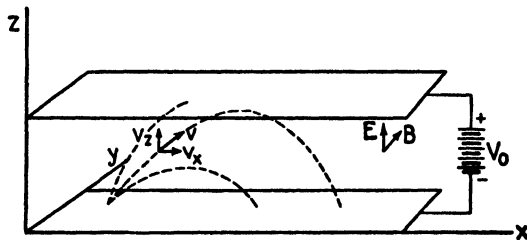
FIG. 6.—Parallel-plane magnetron.
