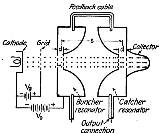
FIG. 10.—Klystron oscillator.
