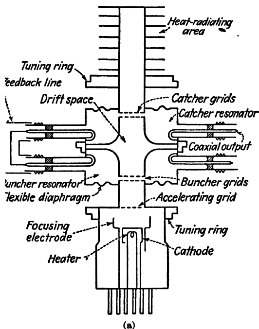
FIG. 5.—Double-resonator klystron.
