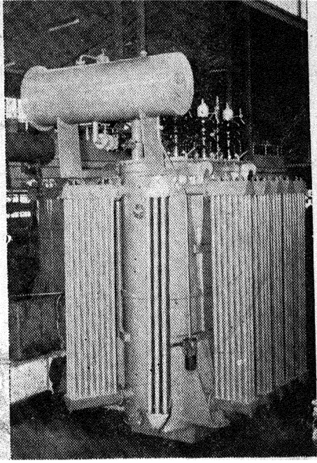
3 M. V. A. ಸಾವರಿನ ಟ್ರಾನ್ಸಫಾರ್ಮರ್ 33/11 K. V.
