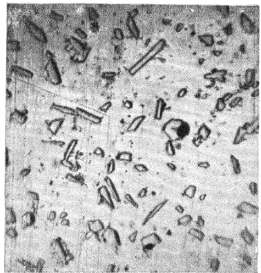
Abb. 11 Künstlicher Rabbit, Legierung mit 10% Ni + 2% P, 30 h auf 800^\circ erhitzt 300 × vergrößert
