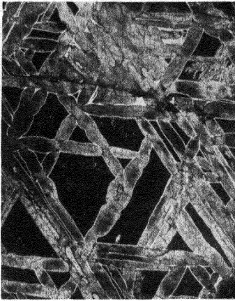
Abb. 1 Widmannstättensche Struktur (Brückwasser) 4 \times vergrößert
