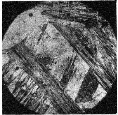
Abb. 8 Zwillingslamellenstruktur (Braunau, \frac{1}{2} h auf 1450^\circ erhitzt, bei 1200^\circ abgeschreckt) 100 × vergrößert
