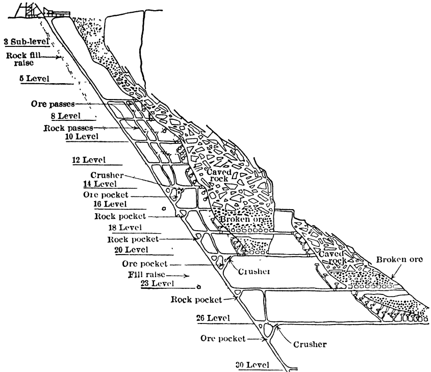
Fig 455. Cross-sec Creighton Mine, Ont
