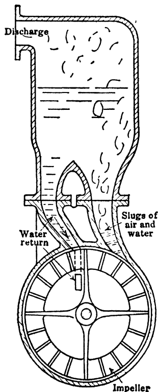
Fig 17. La Bour Pump
