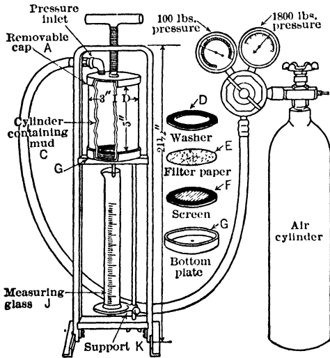
Fig 23. Baroid 100-lb Tester
