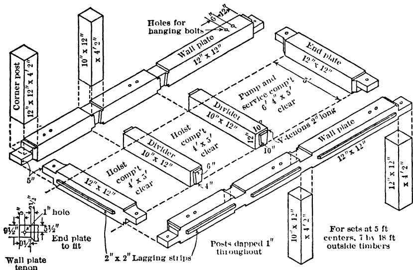
Fig. 21. Shaft Set
