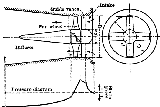
Fig 40 Propeller Fan (7)
