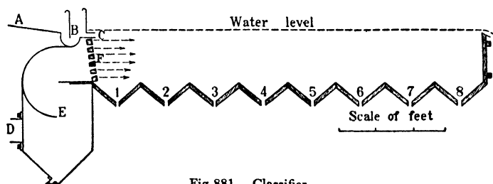
Fig 881. Classifier
