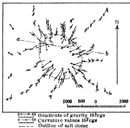
Fig 9. Gravimetric Anomalies due to a Salt Dome (4)
