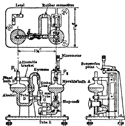
Fig 20. Wahlen Gage (diagrammatic)
