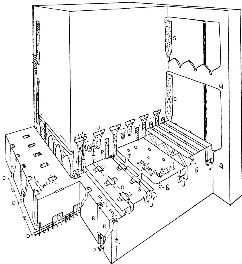
Fig 551. Sublevel Undercut Caving Method, Ray Mine, Ariz (294)
