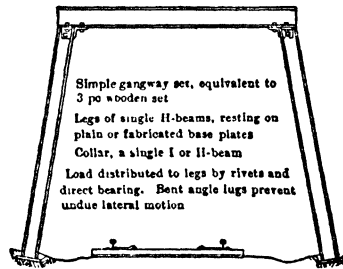
Fig 786. Gangway Set, Style F
