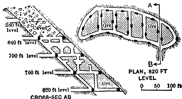
Fig 217 Glory-hole Mining, Marquette Range, Mich
