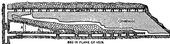
Fig 436. Shrinkage Stope, Coniagas Mine, Cobalt, Ont
