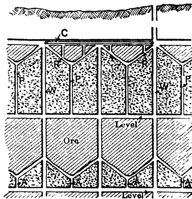
Fig 413. Rill Stopes, Kalgoorlie
