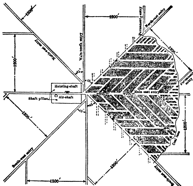
Fig 766. Longwall Mine
