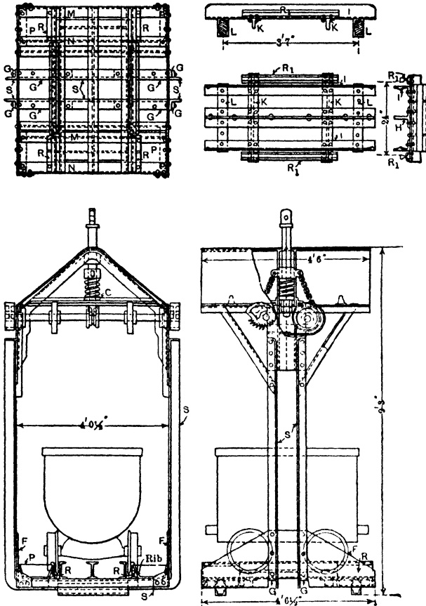
Fig 118. Drop-bottom Cage
