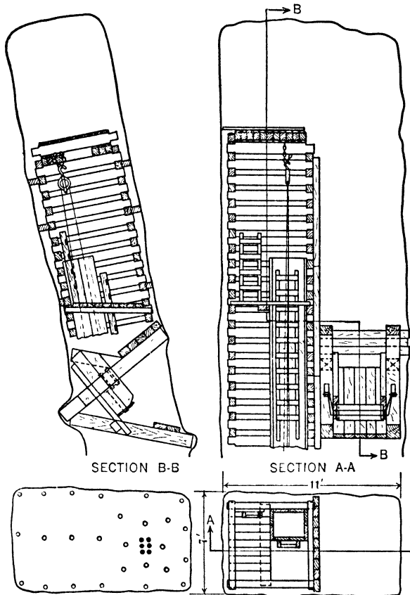
Fig 164. Plan and Sec of Fill Raise, Frood Mine, Ont
