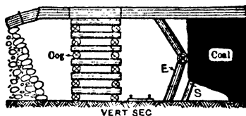
Fig 763. Longwall Face
