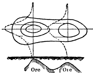
Fig 24. Example of Equipotential Curves (9)
