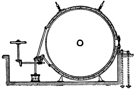
Fig 17. Band Brake
