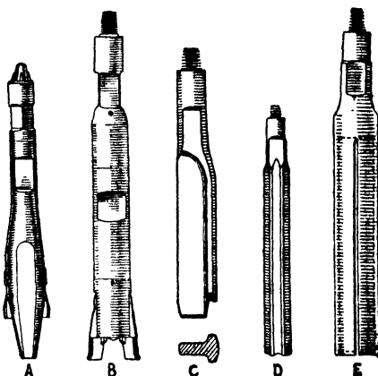
Fig 18. Reamers
