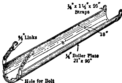
Fig 652. Shaking Chute
