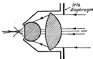
Fig. 41.—Abbe Condenser
